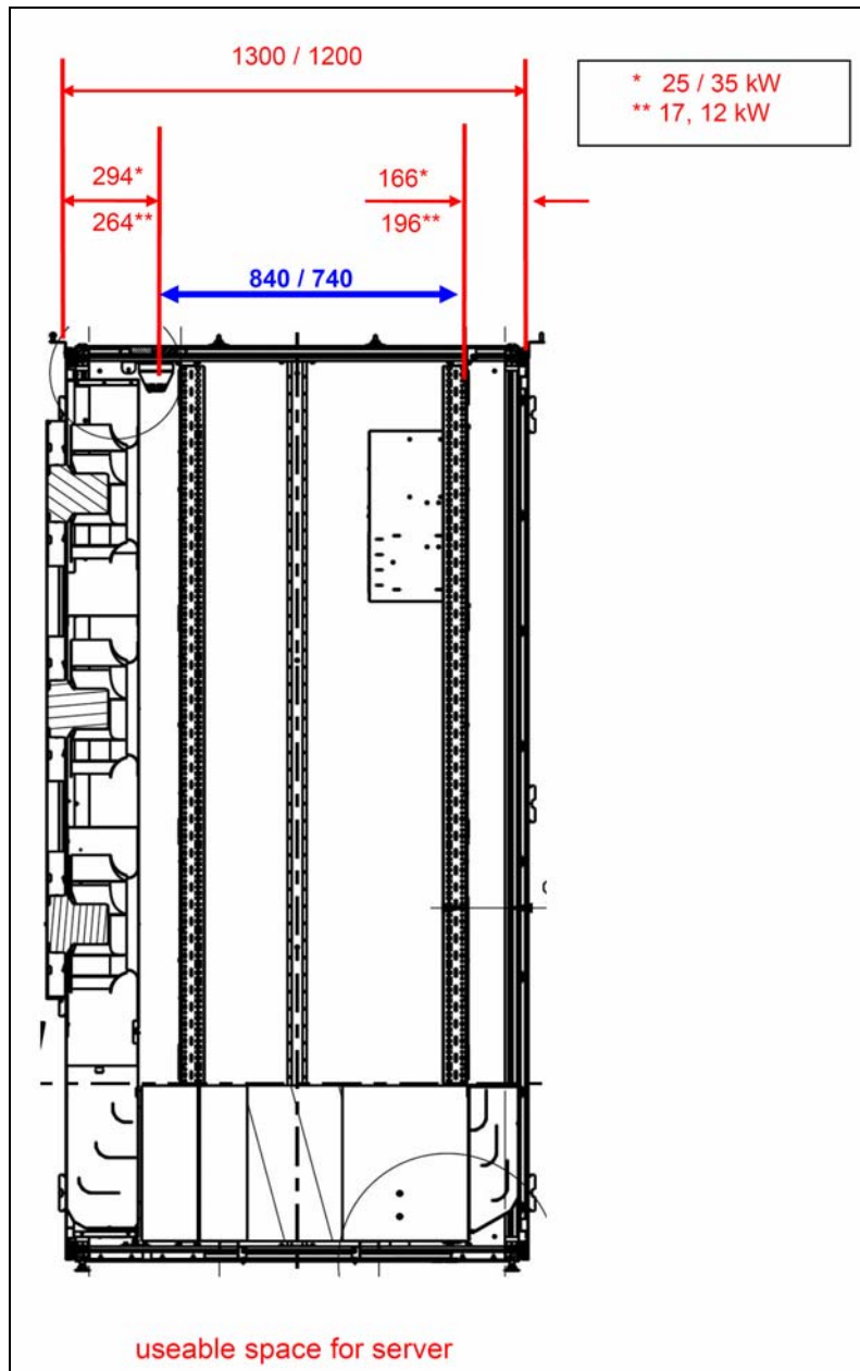
Nutzbare Länge für Server / Einbauten
